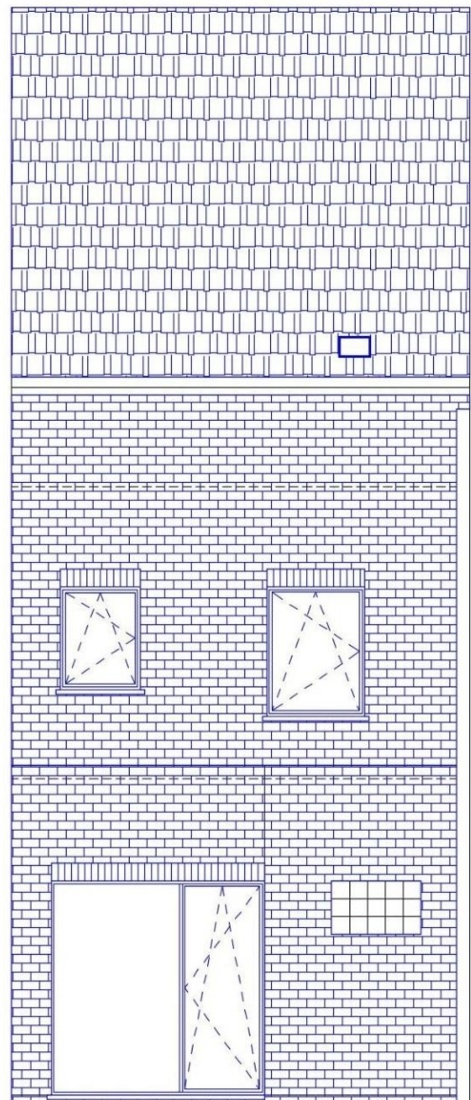
Ontworpen Achtergevel
